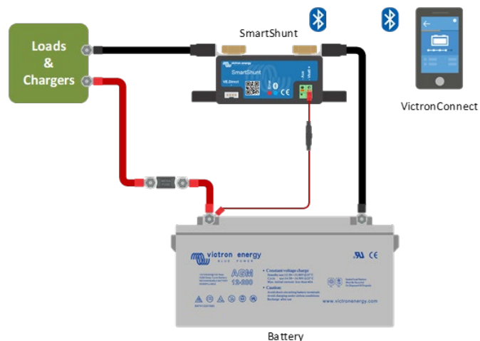
Cabos básicos do SmartShunt
